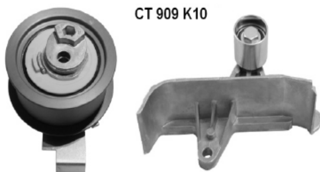
Рис. 2 Новая система натяжения
